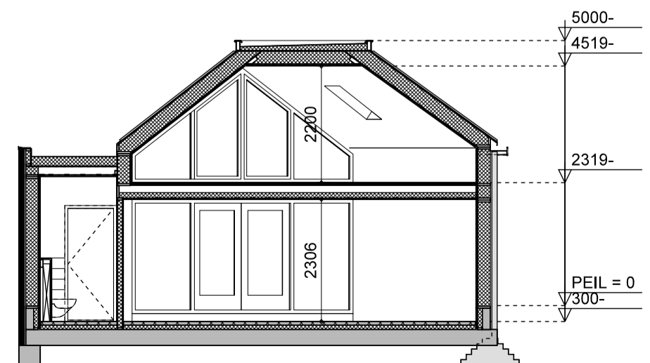
Doorsnede 1:100
